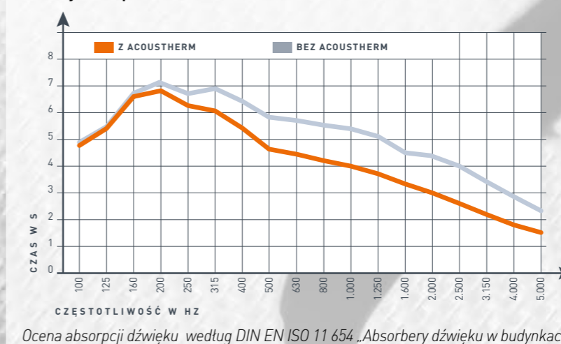
Redukcja echa przez zastosowanie SYSTEXX Active AcousTherm
